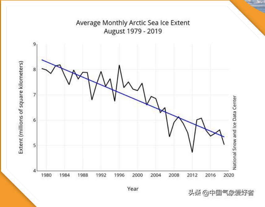
1979~2019 北極浮冰量
